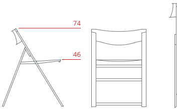
Sedia pieghevole 1PO5511 : L 52 P 58 H 74
