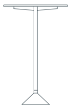
Side table 1TU6521: Ø 15¾ H 24½
