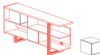
1VR3510/11: L 250 P 55,5 H 106,5 *1VR3610: L 48,5 P 43 H 37
