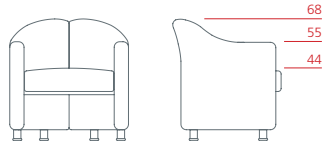
Poltroncina bassa su piedini 1PS6012: L 68 P 60 H 68
